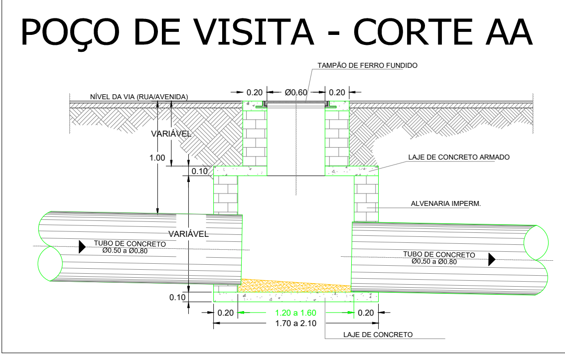
DETALHE DA POÇO DE VISITA S/ ESCALA
