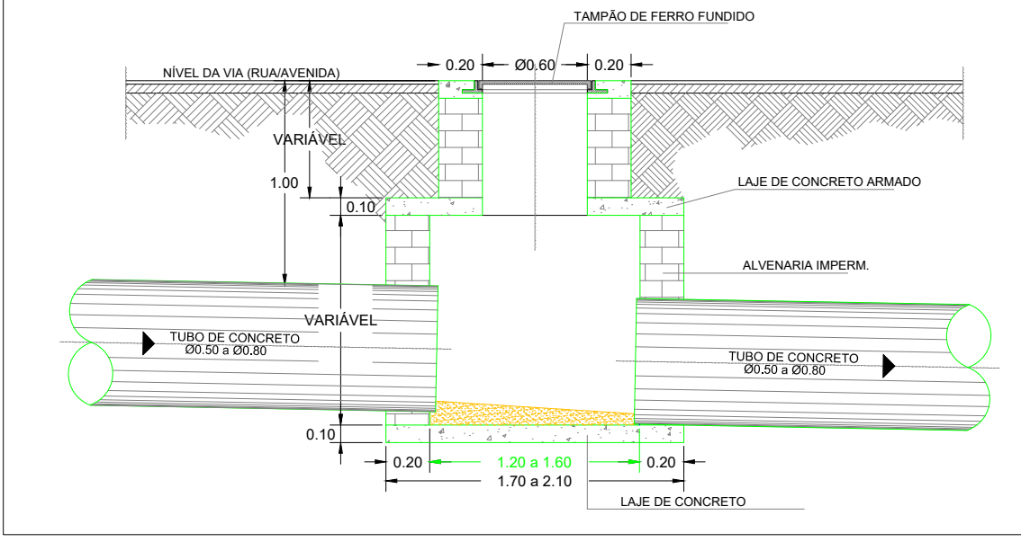
POÇO DE VISITA - CORTE AA
