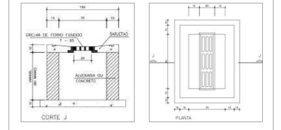
DETALHE DA BOCA DE LEÃO EM CORTE S/ ESCALA DETALHE DA BOCA DE LEÃO EM PLANTA S/ ESCALA
