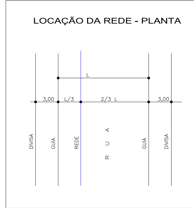
DETALHE DA LOCAÇÃO DA REDE S/ ESCALA
