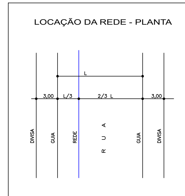
DETALHE DA REDE DE DRENAGEM S/ ESCALA
