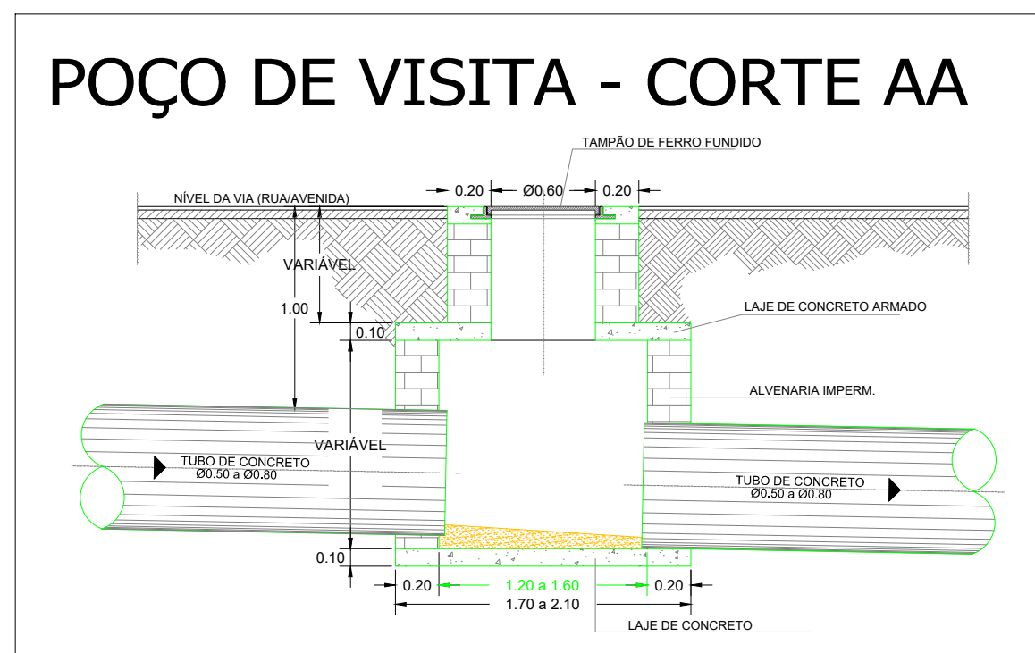
DETALHE DA POÇO DE VISITA S/ ESCALA
