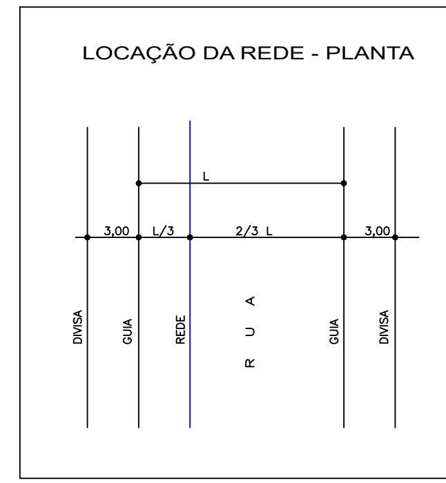
DETALHE DA REDE DE DRENAGEM S/ ESCALA
