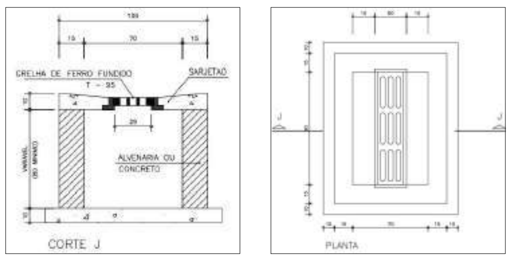
DETALHE DA BOCA DE LEÃO EM CORTE S/ ESCALA DETALHE DA BOCA DE LEÃO EM PLANTA S/ ESCALA
