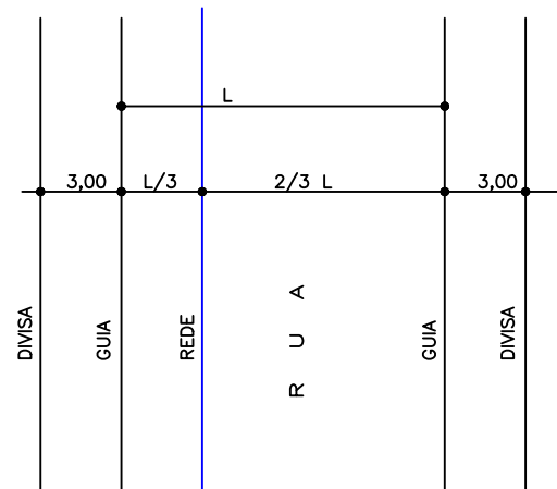
LOCAÇÃO DA REDE - PLANTA
