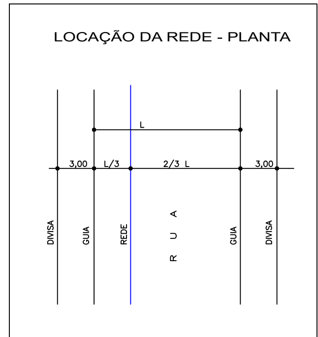
DETALHE DA LOCAÇÃO DA REDE S/ ESCALA
